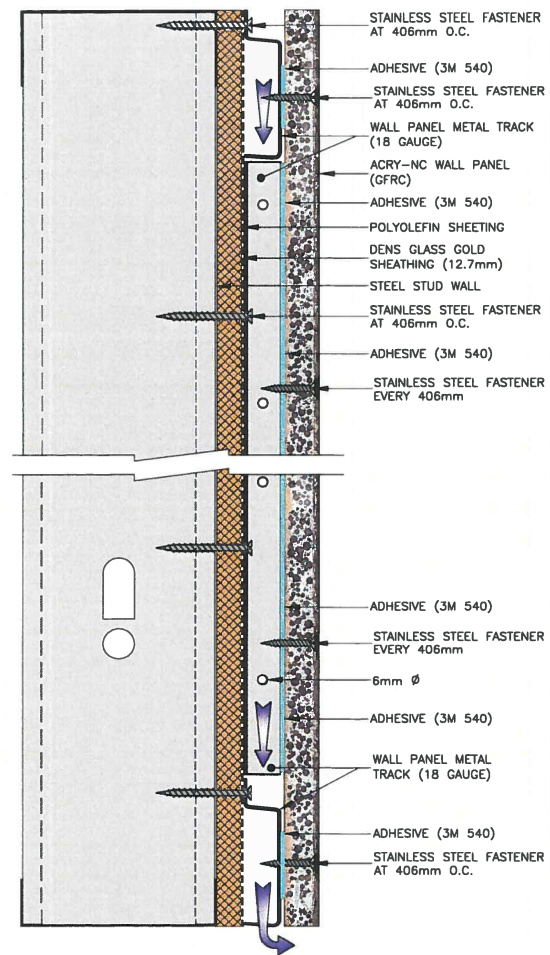
① WALL SECTION Scale: 1:2.5
